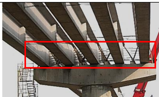
照片 6：吊放後-斜撐只於兩端帽梁
